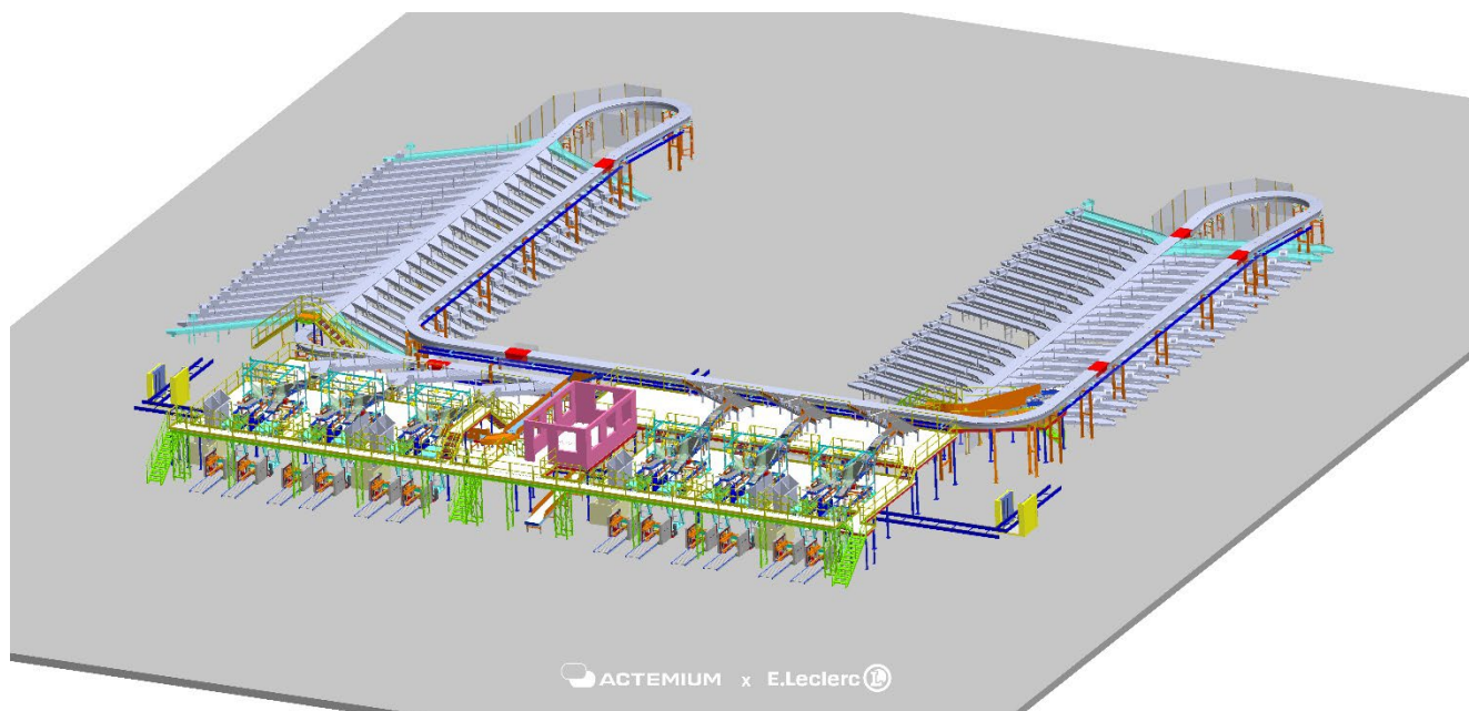
Vue 3D de l'installation Scacentre par Actemium Lyon Logistics
